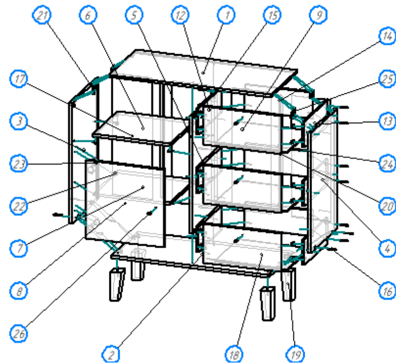
Рис.1 Сборка корпуса
